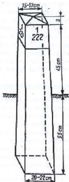
Betonowy słup oddz. z numeracją według obrzeźbów
